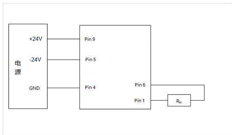
图11 MCT3000接线图
