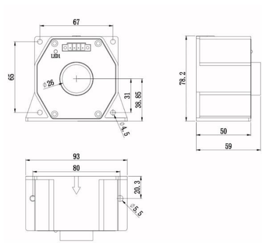
图 3 MCT200 外形图
