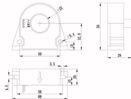
图 1 LCT200 外形图
