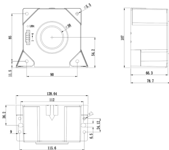
图 4 MCT500、MCT1000 外形图
